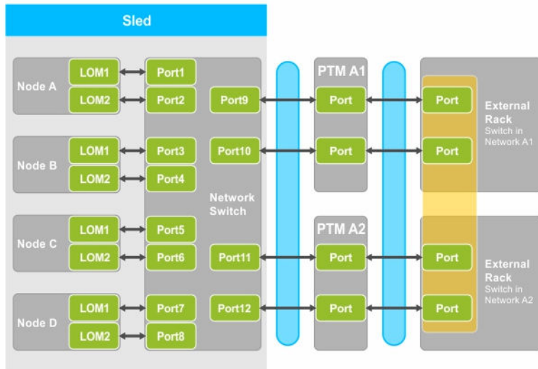
図 5. 標準構成
