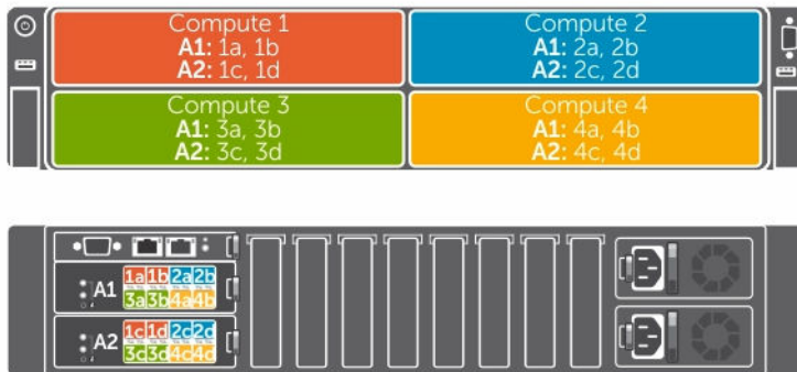
図 9. 拡張ネットワーク分離構成用のパススルーモジュールポートマッピングへのノード
